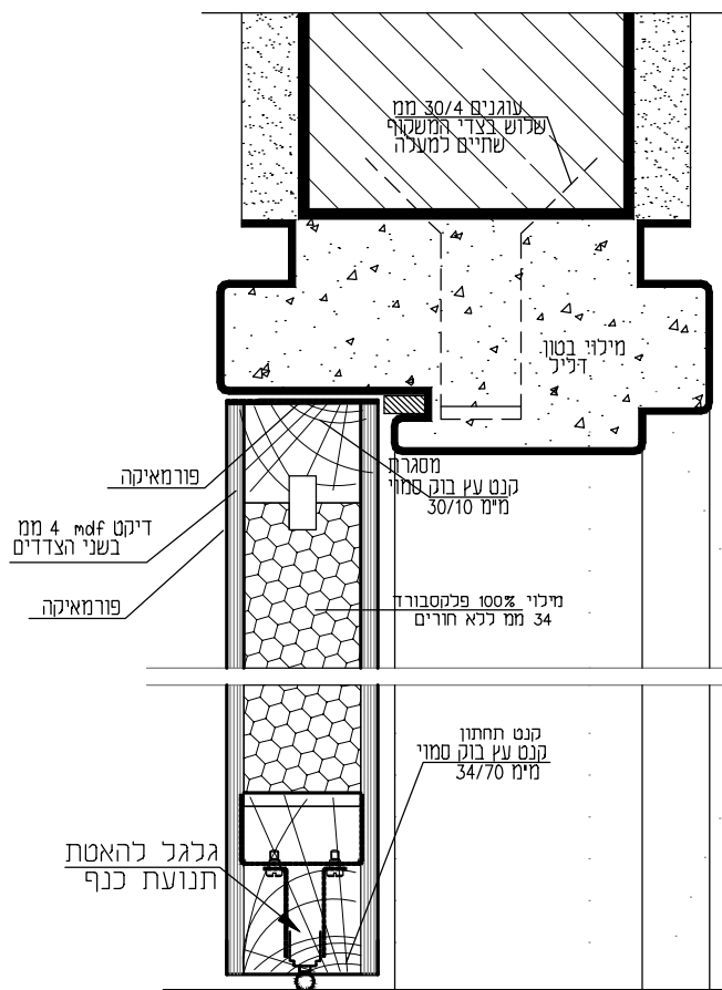
פרט דלת קנ"מ 1:2.5
