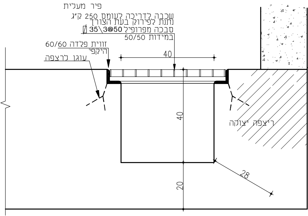
פרט 4 פיר מעלית קנ"מ 1:10
