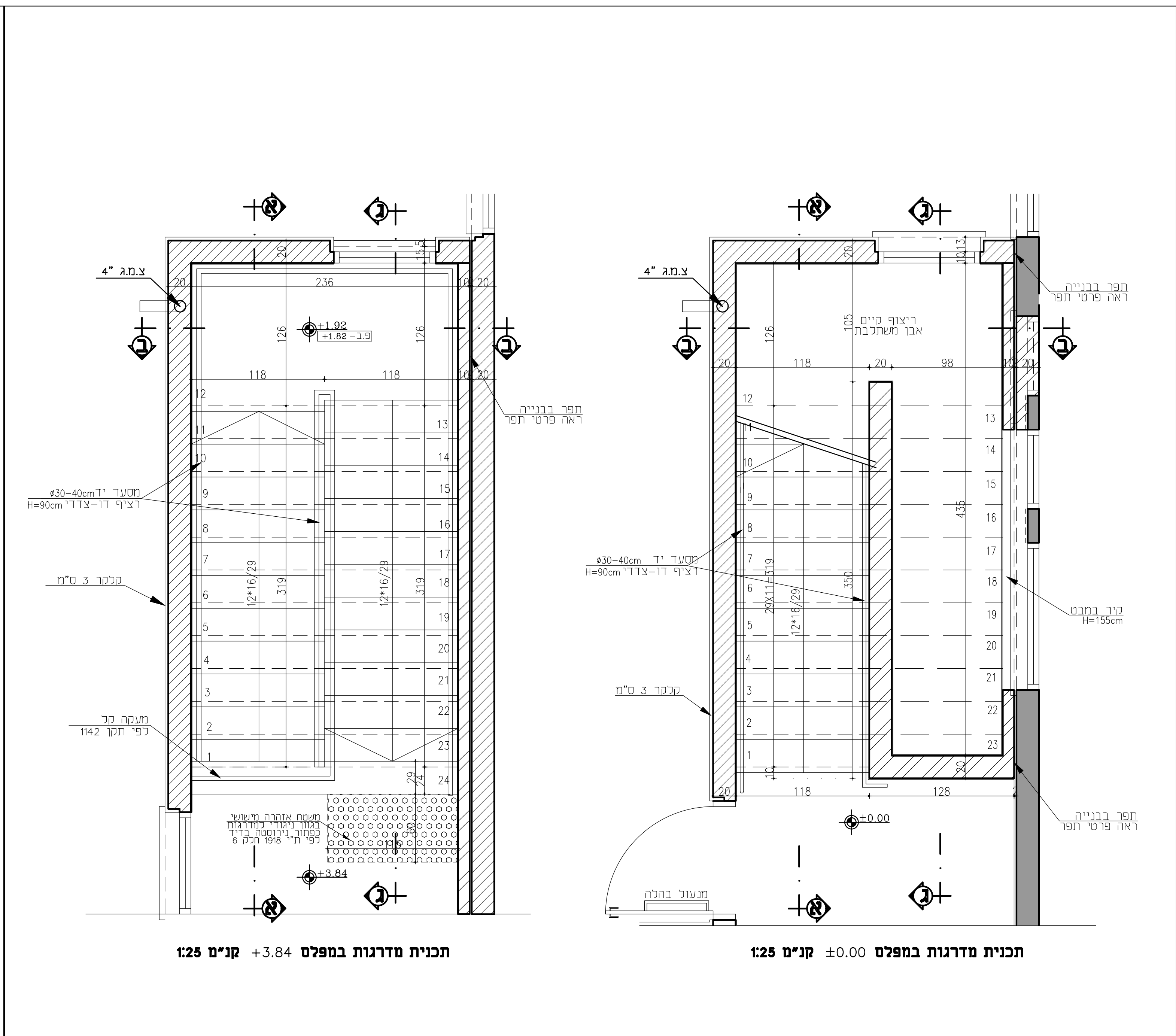
קנה מידה 1:10 פרטי מדרגות קנה מידה 1:25 תכנית מדרגות פנים
