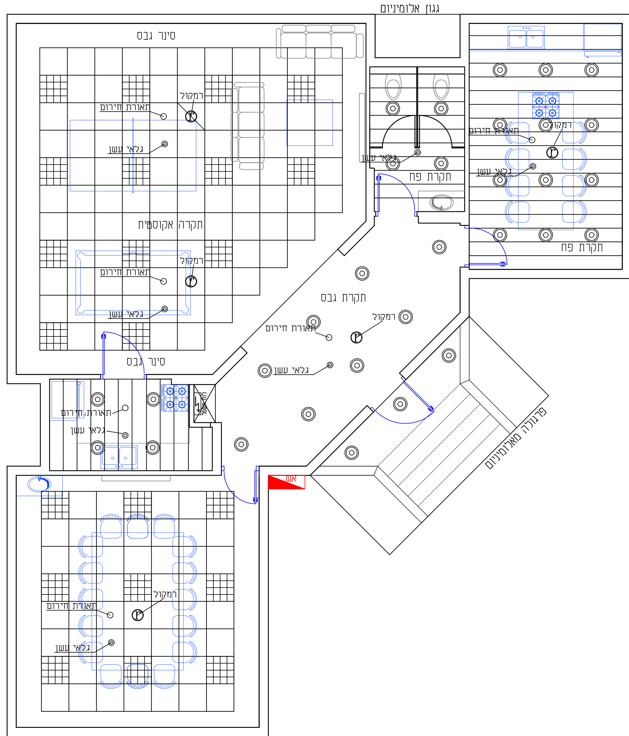
תוכנית תקרה ותאורה קנה מידה 1:50
