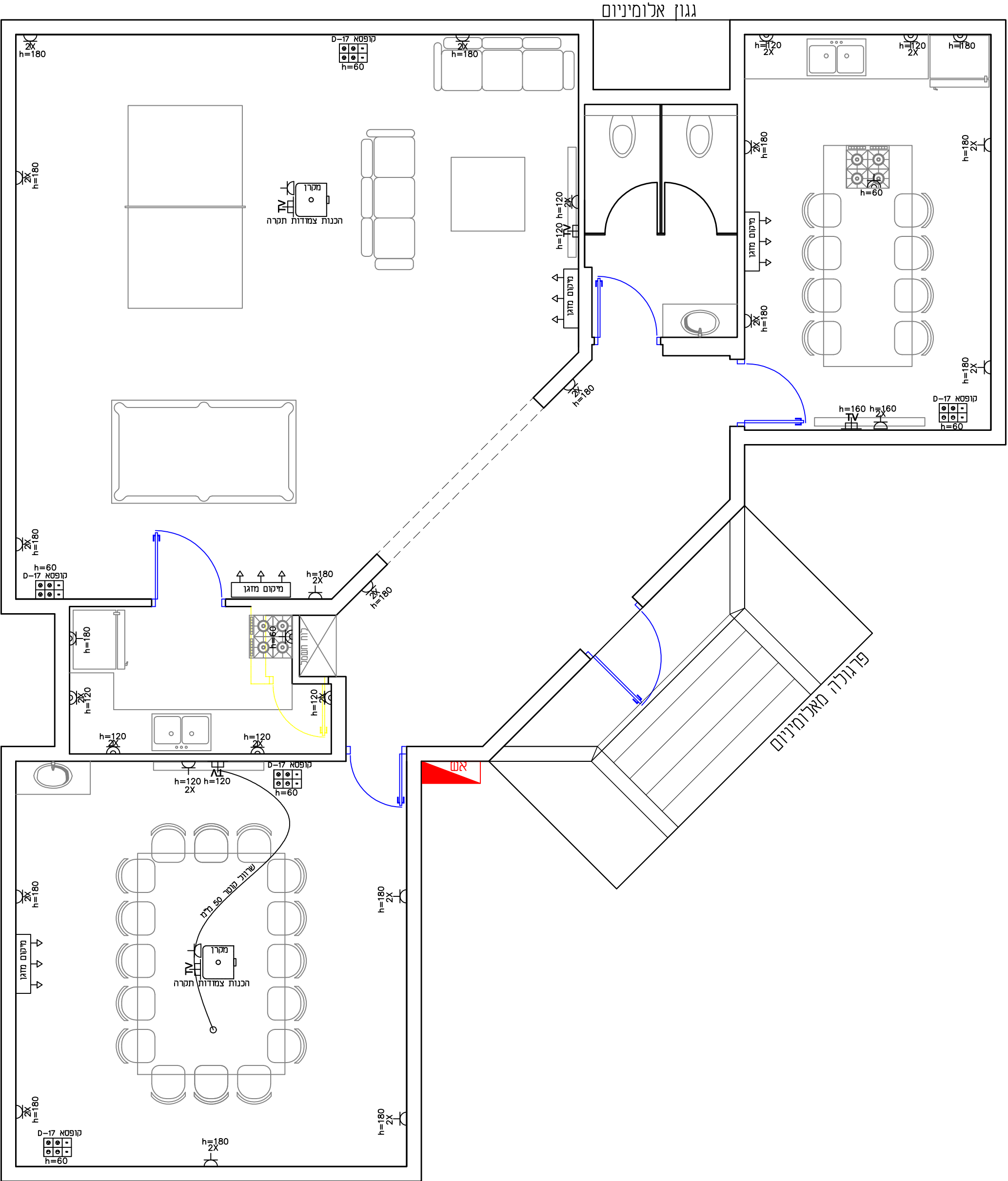
תוכנית מיקום נקודות חשמל קנה מידה 1:50
